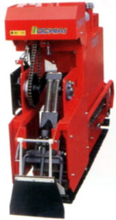
深耕・中耕装置 OMT-D1
